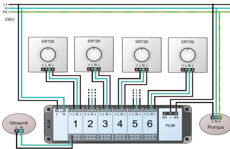
Сервомотор Каждая секция подключение к 4 сервомоторам Насос
