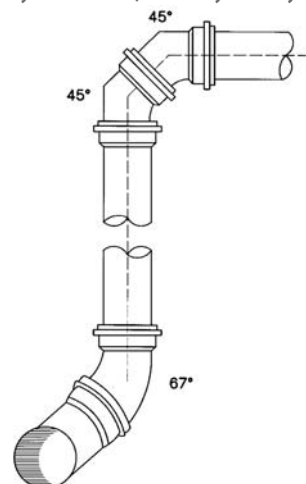
Рис. 12 Пример вертикального подключения к главному канализационному каналу
