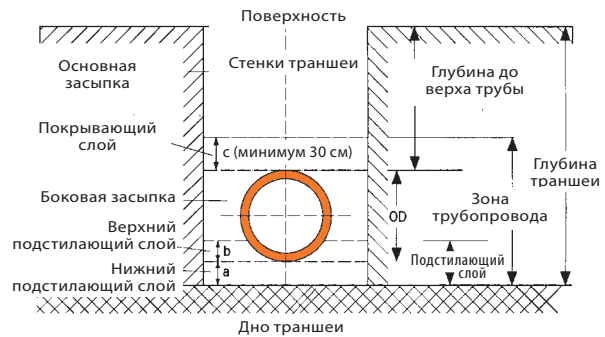
Рис. 3 Устройство траншеи
